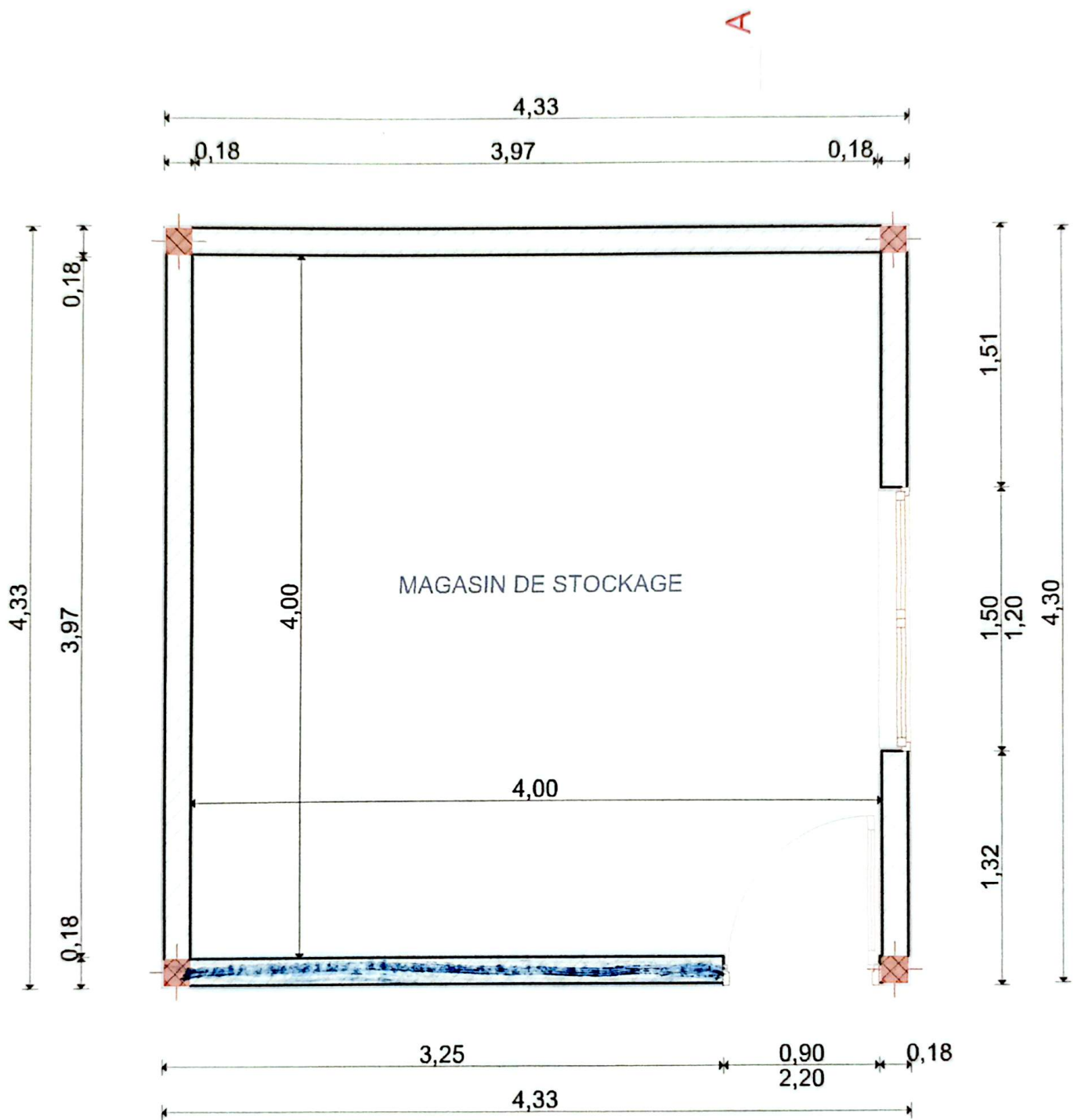
PLAN DE DISTRIBUTION A Ech 1:50e
